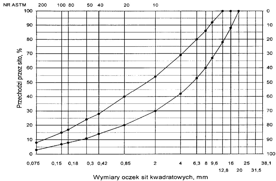
Rys. 5. Krzywe graniczne uziarnienia mieszanki mineralnej BA od 0 do 16 mm do warstwy wiążącej, wyrównawczej i wzmacniającej nawierzchni drogi o obciążeniu ruchem KR1 lub KR2
